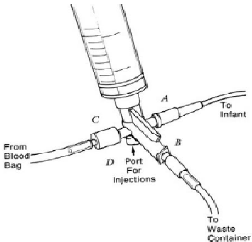
Gambar 16. Katup 4-arah.
